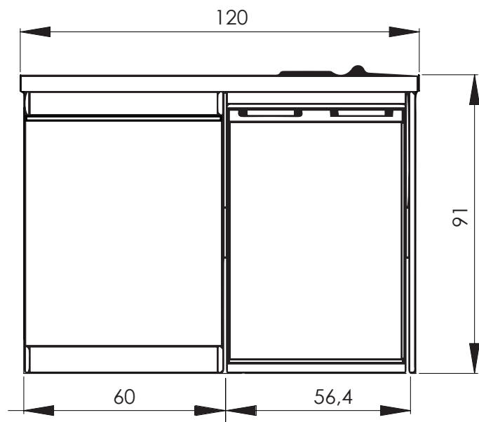
Vue face
